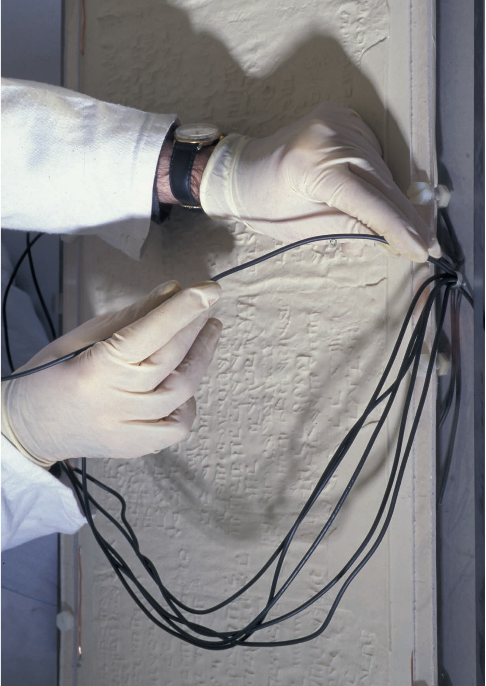
PLANCHE CCLXXXIX Préparation de la cathode – montage des connexions électriques
