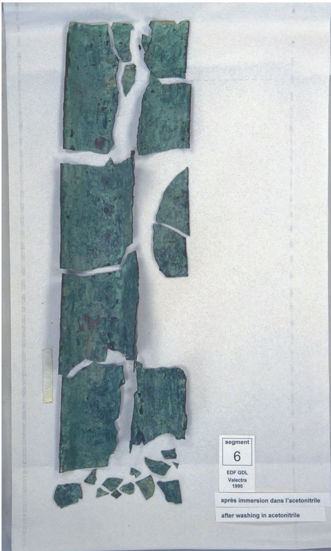
PLANCHE CCLXIX Segment 6 après immersion dans l'acetonitrile (recto)
